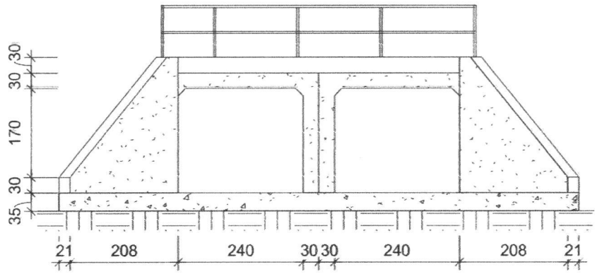
2 VISTA LATERAL 1 : 100
