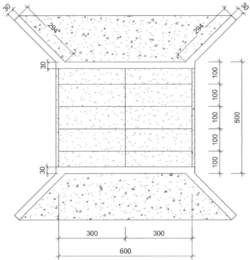
1 PLANTA BAIXA 1 : 100
