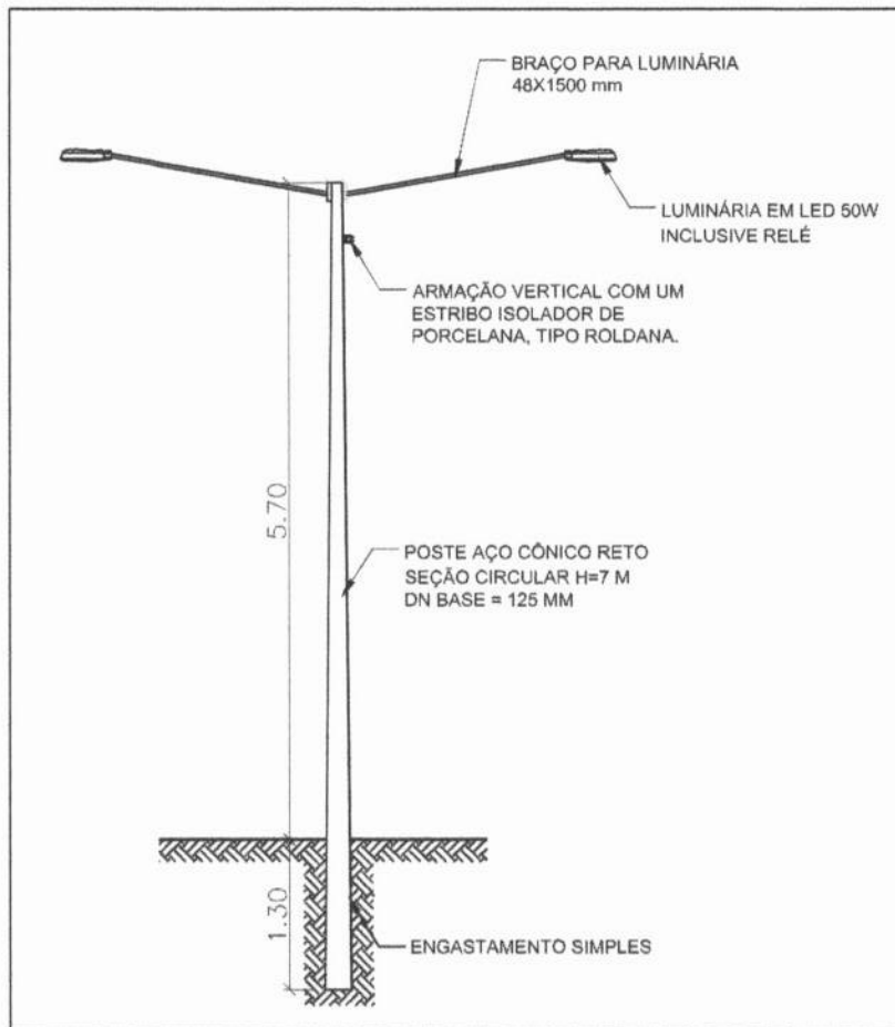
01 DET. POSTE DE ILUMINAÇÃO 005 ESCALA 1:50
