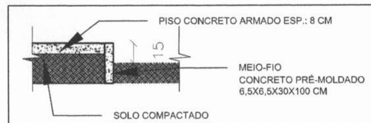
02 DET. MEIO-FIO E PISO 005 ESCALA 1:20
