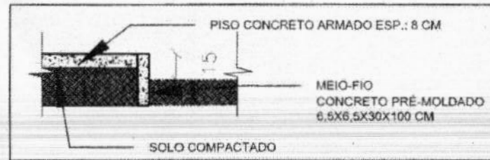
02 DET. MEIO-FIO E PISO 005 ESCALA 1:20
