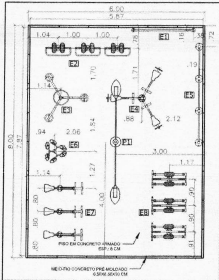
01 PLANTA BAIXA 004 ESCALA 1:50
