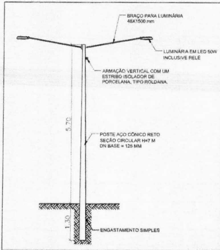
01 DET. POSTE DE ILUMINAÇÃO 005 ESCALA 1:50
