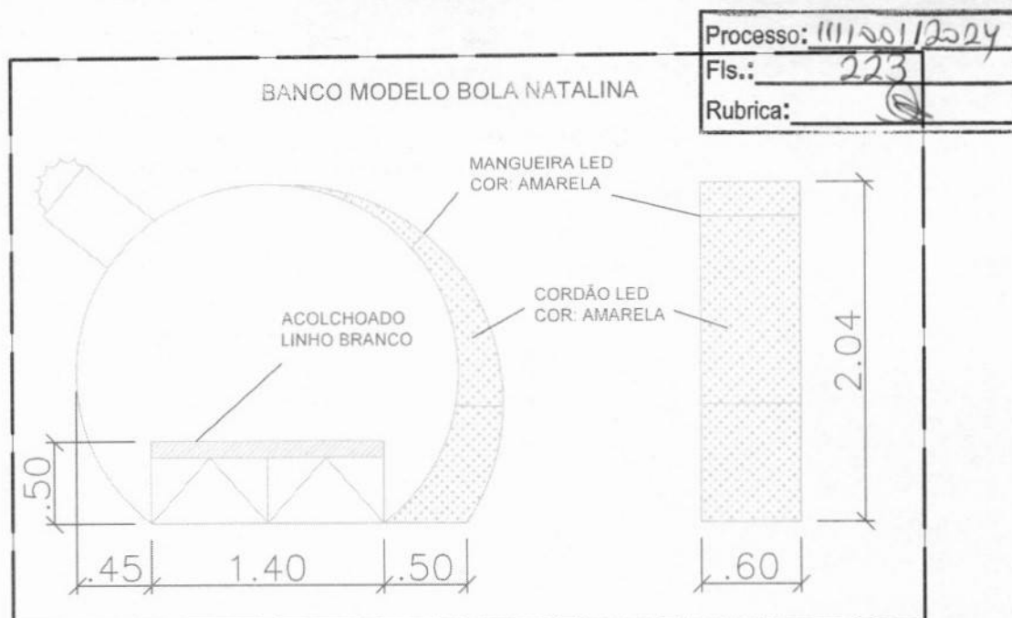
Banco Modelo Bola Natalina (03 unidades) (Medidas em Metros)
