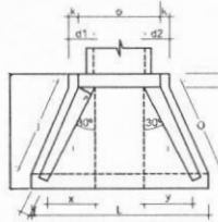
PLANTA NORMAL - SIMPLES
