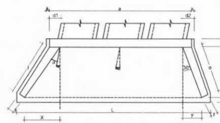
PLANTA ESCONSA - TRIPLO
