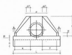
VISTA FRONTAL - SIMPLES
