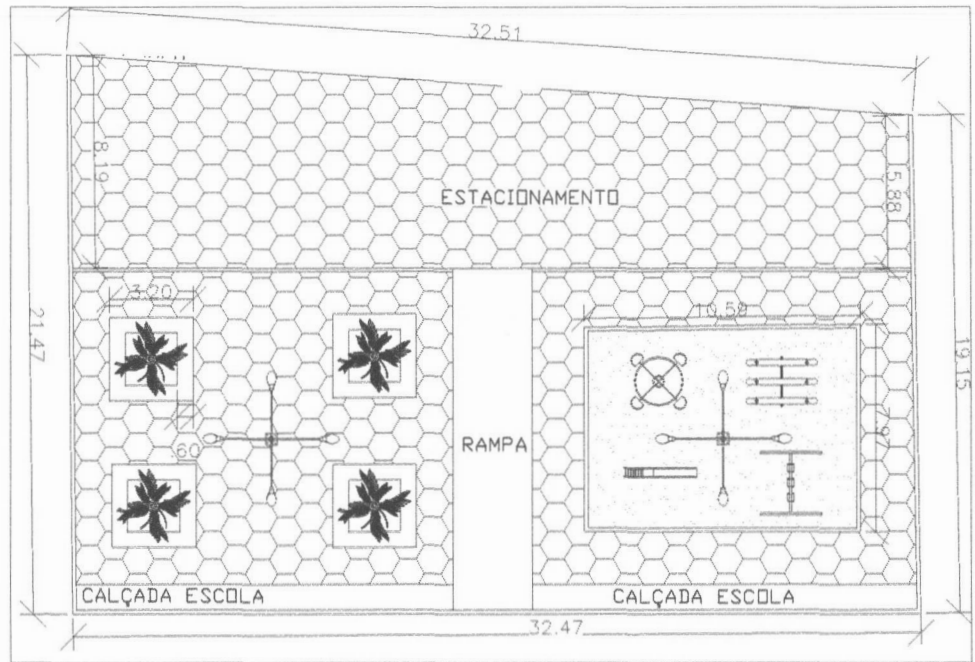
6 AMPLIÇÃO - PRAÇA ESC: 1:100
