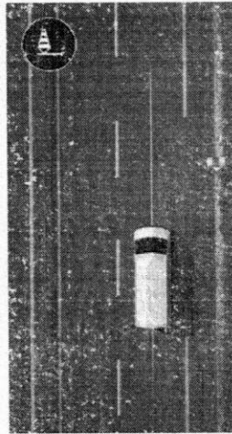
controle de estabilidade (ESP) e controle adaptativo de carga (LAC) O ESP corrige a trajetória do carro para evitar derrapagens. O controle adaptativo de carga identifica o deslocamento da carga e o centro de gravidade do veículo para otimizar a eficiência da frenagem, o tração e a estabilidade.
